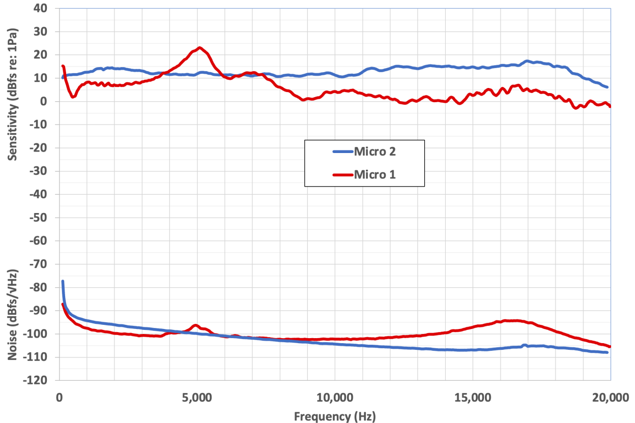
Figura 2. Sensibilidad y umbral mínimo de ruido del Song Meter Micro 1 y del Song Meter Micro 2
