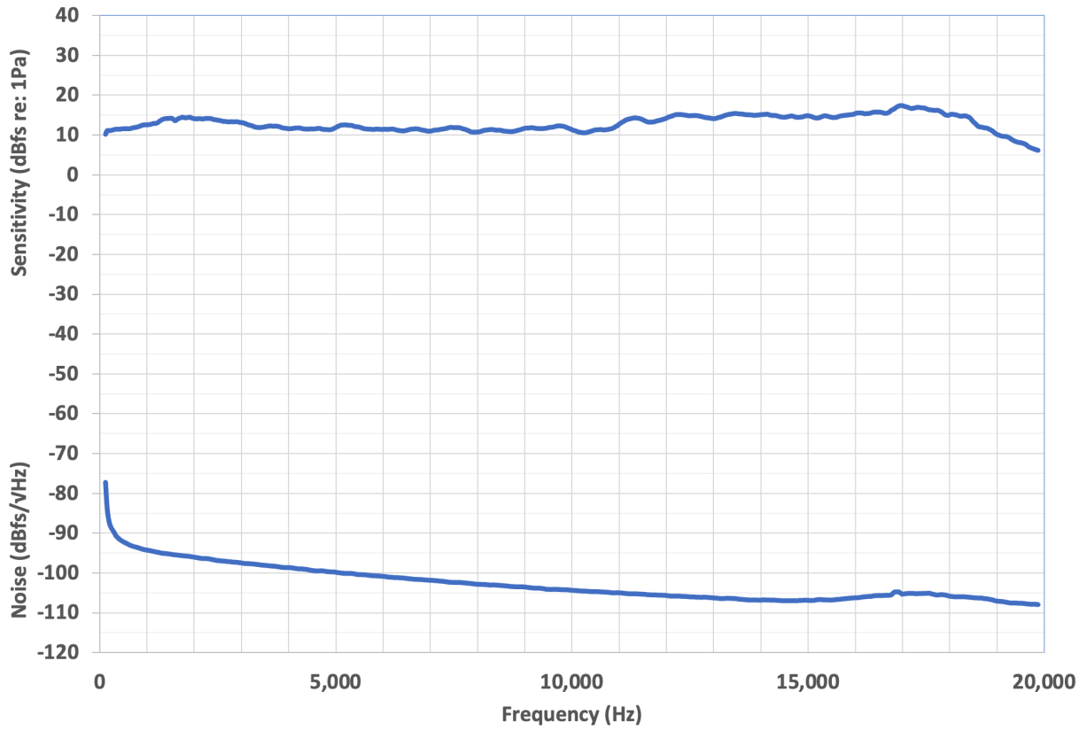
Figura 8. Sensibilidad y umbral mínimo de ruido, escala de frecuencia lineal
