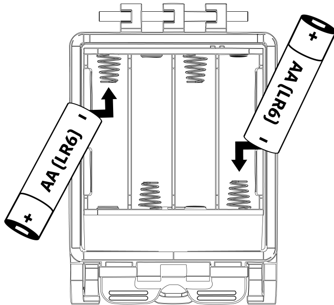
Figura 1. Instalación correcta de las pilas AA
