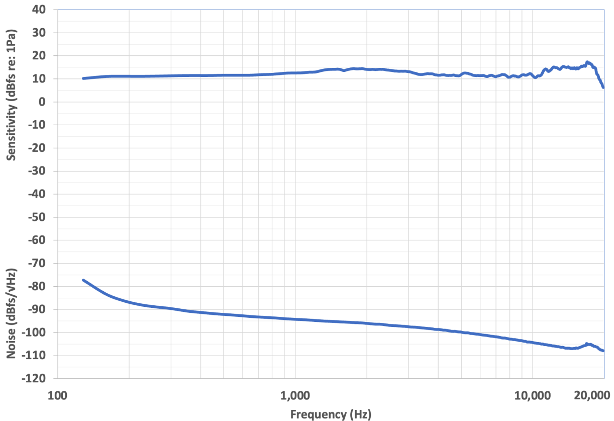
Figura 9. Sensibilidad y umbral mínimo de ruido, escala de frecuencia logarítmica
